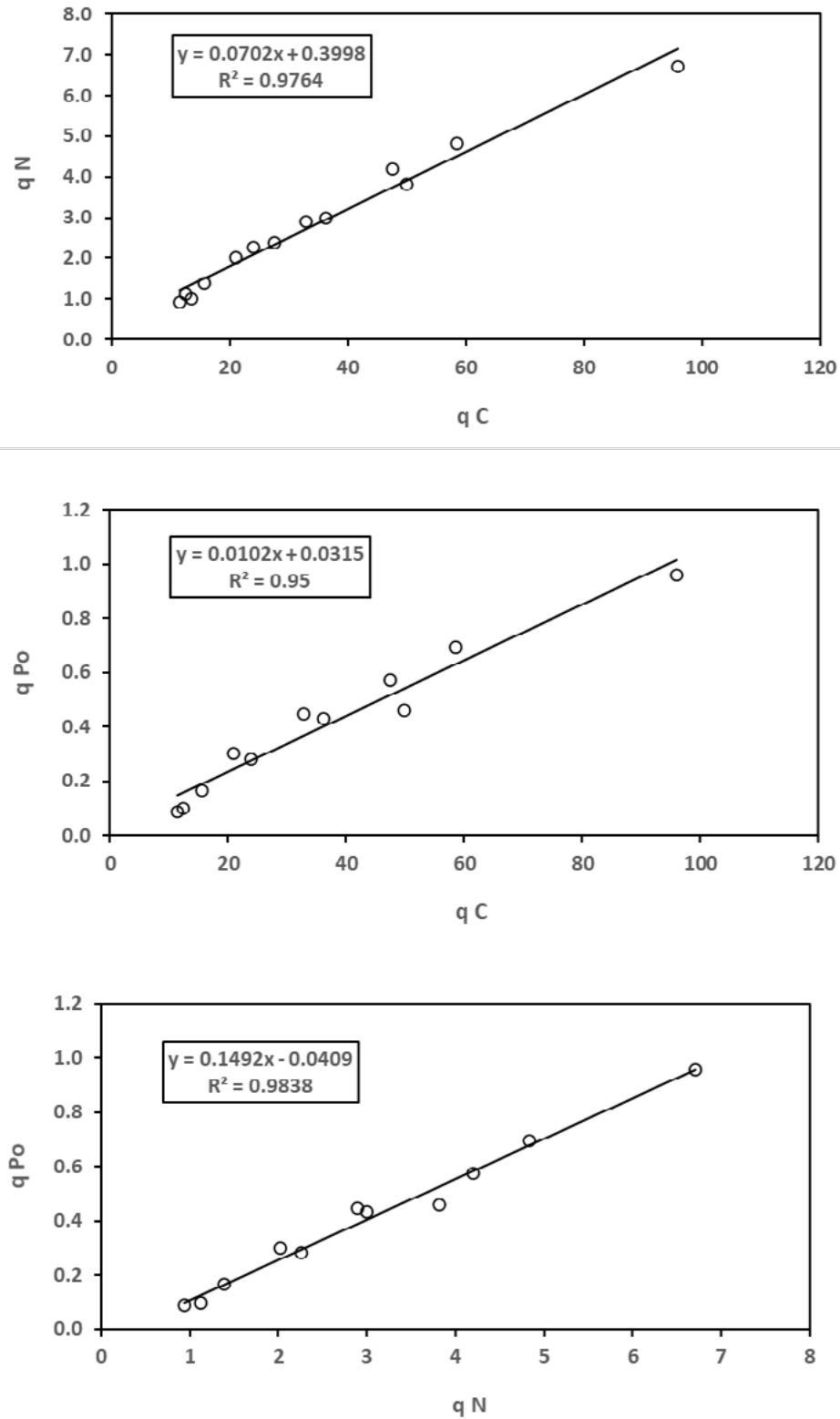
Figura 7. Relaciones entre las pendientes q del modelo COLPOS entre diferentes elementos.
