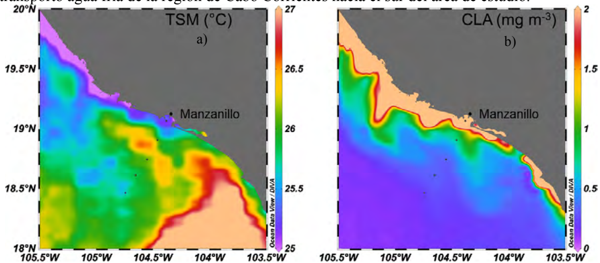
Figura 3. a) Composición promedio satelital de la TSM y b) CLA obtenida de los días del 04 al 11 de abril de 2019.
