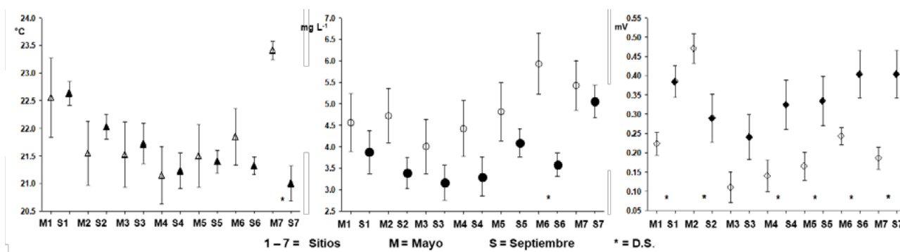
Figura 2. Promedios comparativos intraanuales de Temperatura (°C), OD (mg L -1 ) y POR (mV) entre secas y lluvias. * diferencias significativas con t student.
