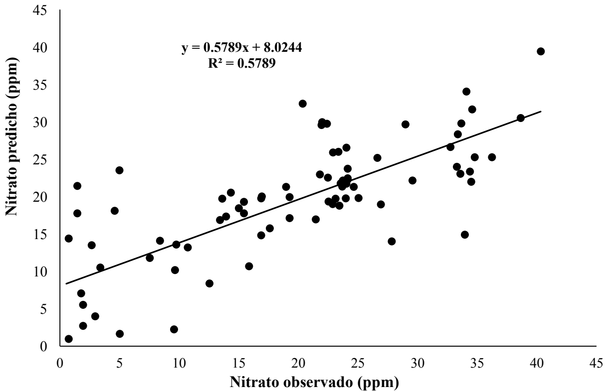
Figura 3. Validación cruzada entre las observaciones de nitratos y lo predicho por la regresión espacial con retraso.
