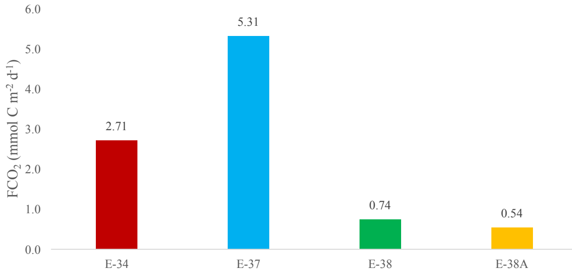
Figura 4. Flujos de \text{CO}_2 océano-atmósfera para el área de estudio del 20 al 27 de abril de 2017.
