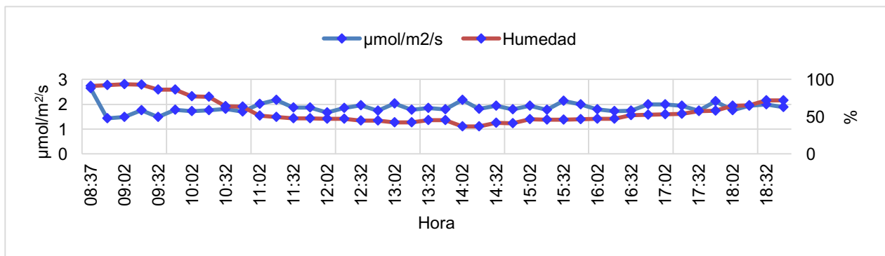
Figura 3. Flujo de CO 2 y humedad del suelo del sitio 1.
