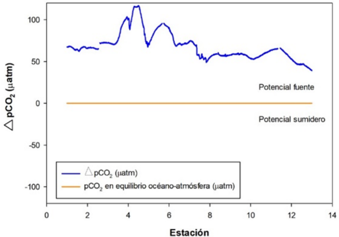
Figura 5. \Delta p\text{CO}_2 calculado ( \mu\text{atm} ) para BLA en agosto del 2018.
