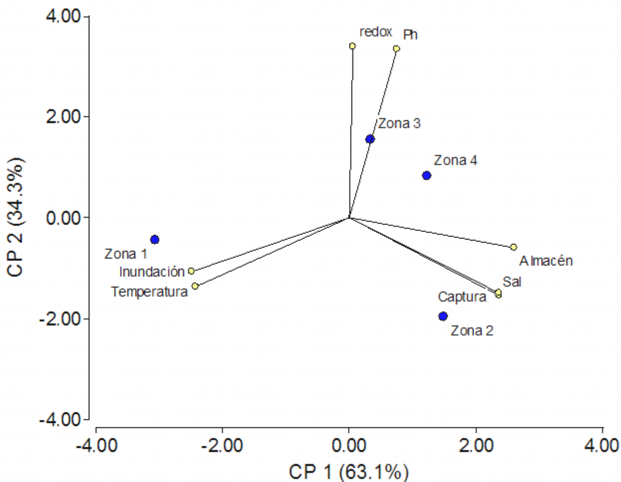
Figura 3. Análisis de componentes principales (ACP) de las variables ambientales, almacén y captura de carbono en la RPMP.
