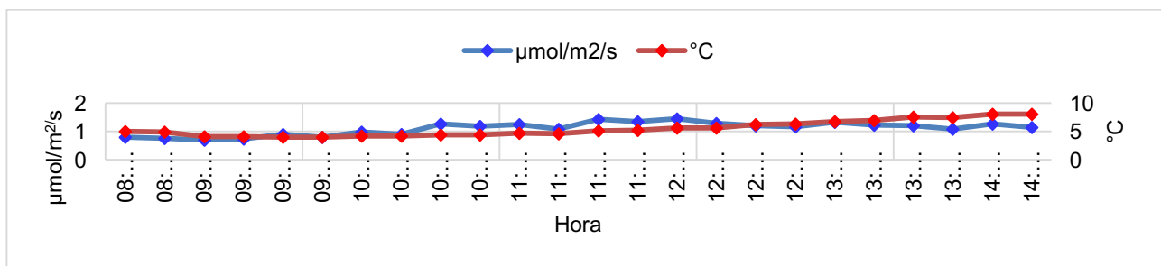
Figura 8. Flujo de CO 2 y temperatura del suelo del sitio 4.
