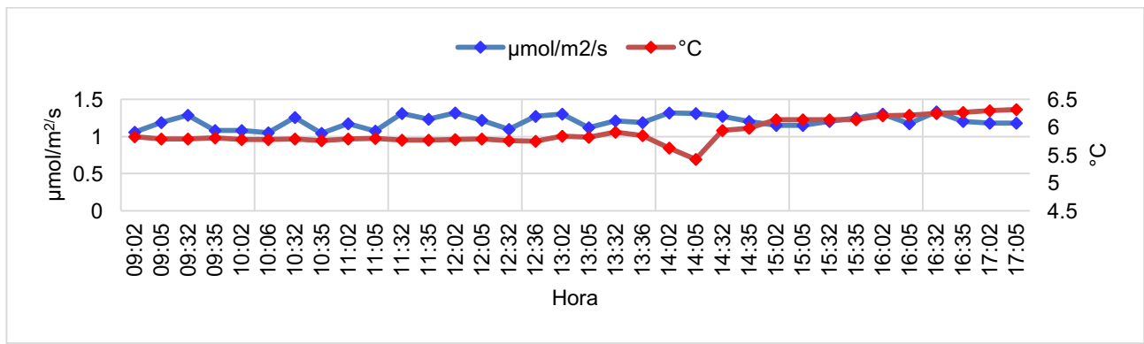
Figura 6. Flujo de CO 2 y temperatura del suelo del sitio 3.
