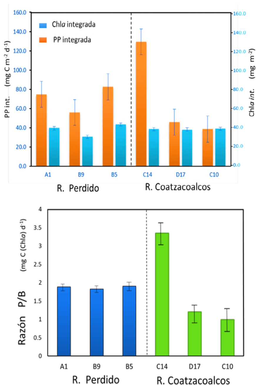
Figura 3. Producción primaria ( \text{mg C m}^{-2} \text{d}^{-1} ) y clorofila a ( \text{mg m}^{-2} ) integradas en la zona eufótica y las razones P/B en estaciones localizadas en las Regiones de Perdido (RP) y Coatzacoalcos (RC) en el Golfo de México durante el crucero Malla Fina -03.
