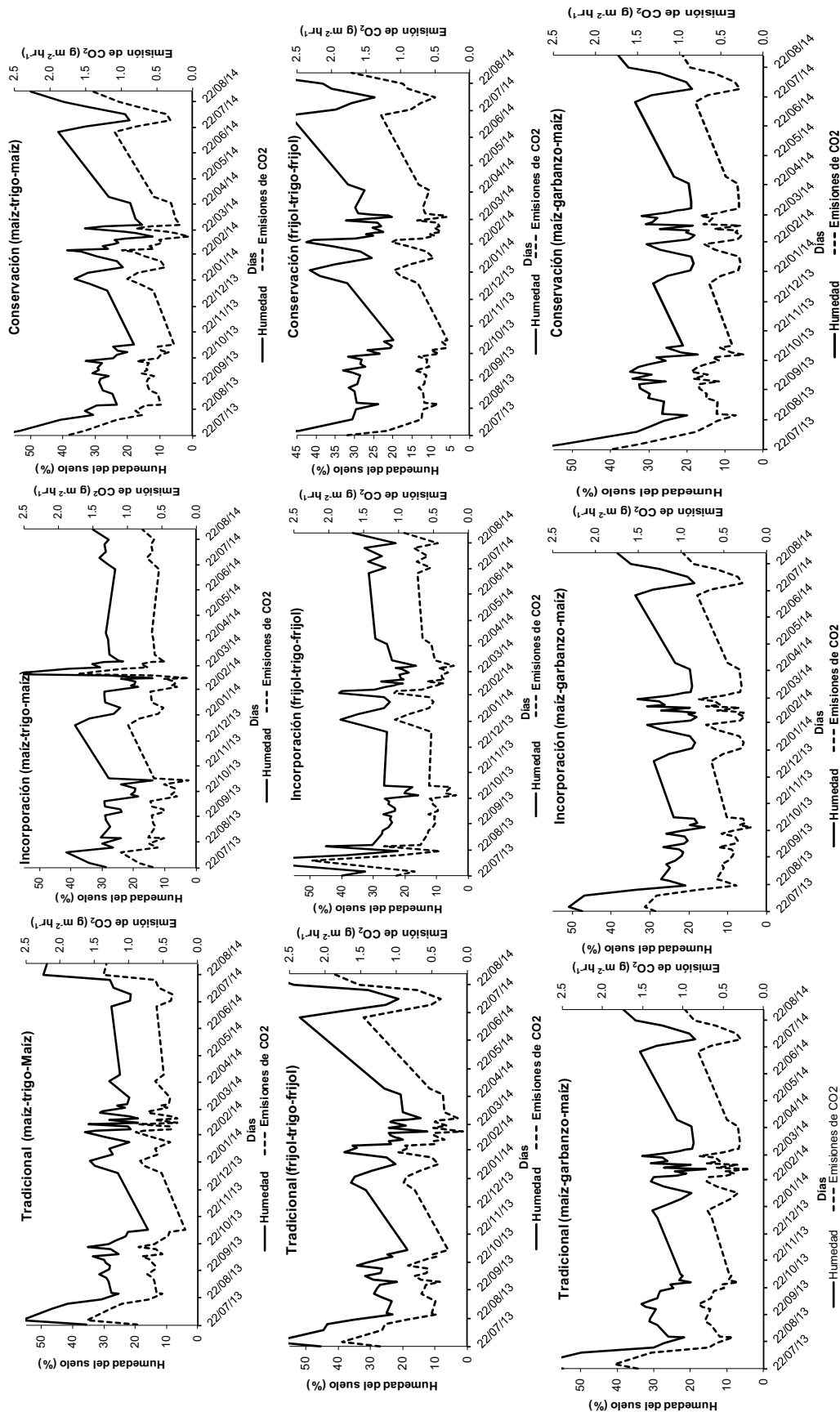
Figura 3. Emisiones de CO 2 en los diferentes sistemas de cultivo de julio de 2013 a agosto de 2014. Campo Experimental Bajío.
