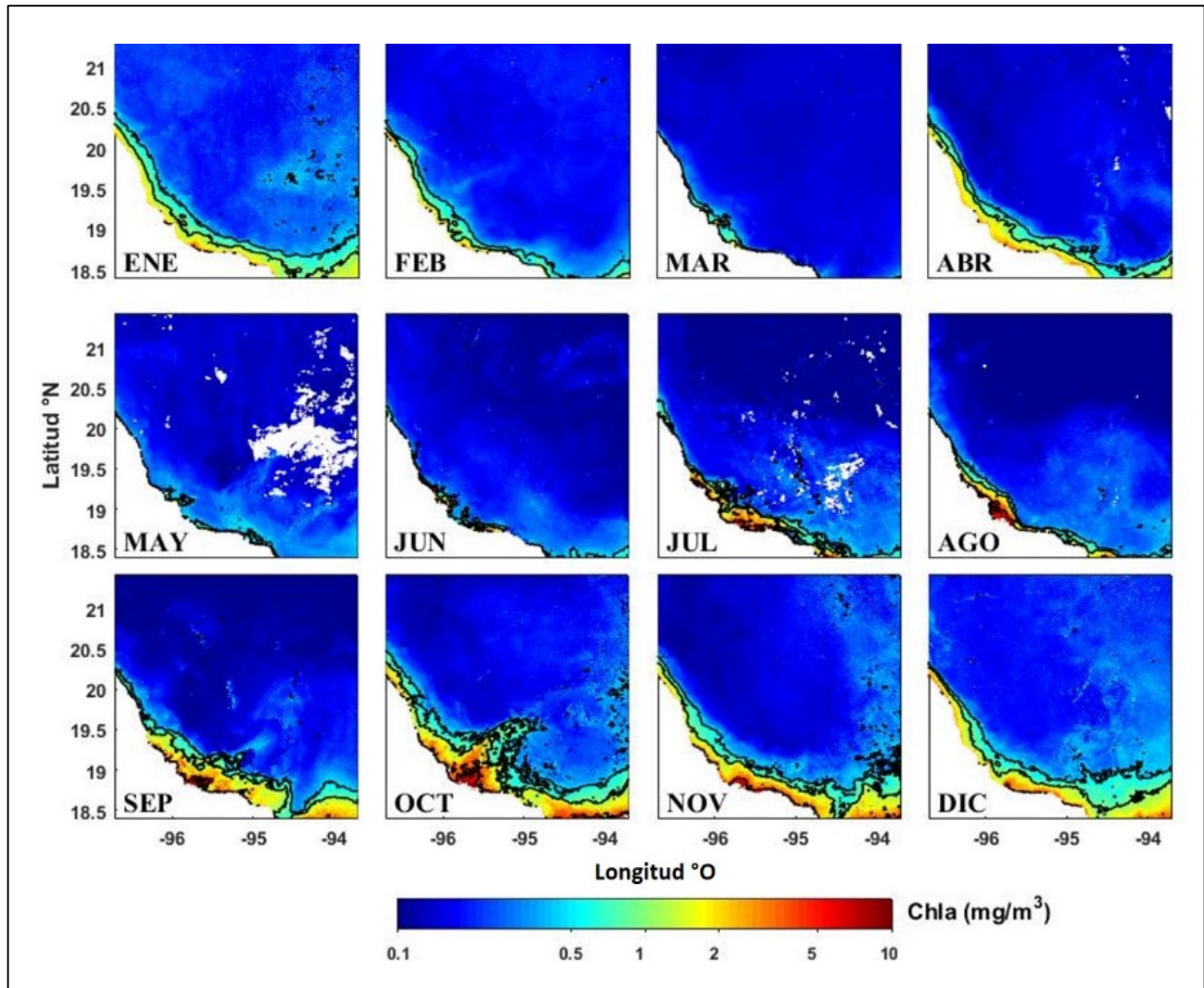
Figura 4. Climatología de la concentración de clorofila-a ( \text{mg}/\text{m}^3 ) frente a costas del centro de Veracruz (2003-2018).
