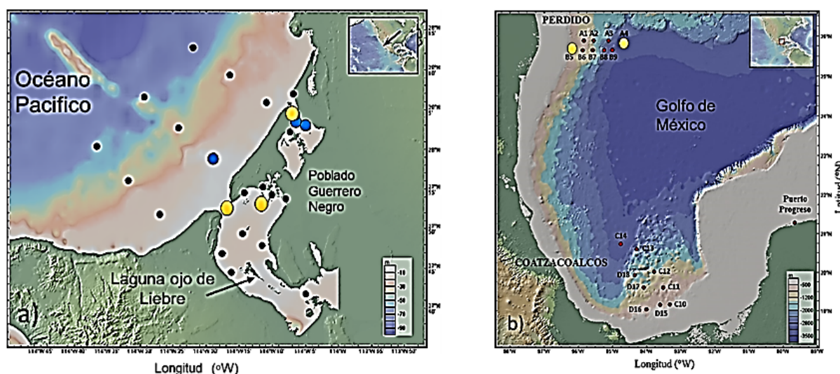
Figura 1. Campañas de muestreo con experimentos de Producción primaria con ^{13}\text{C} ( ^{13}\text{C} -PP). a) Laguna Ojo de Liebre; b) Región Perdido.
