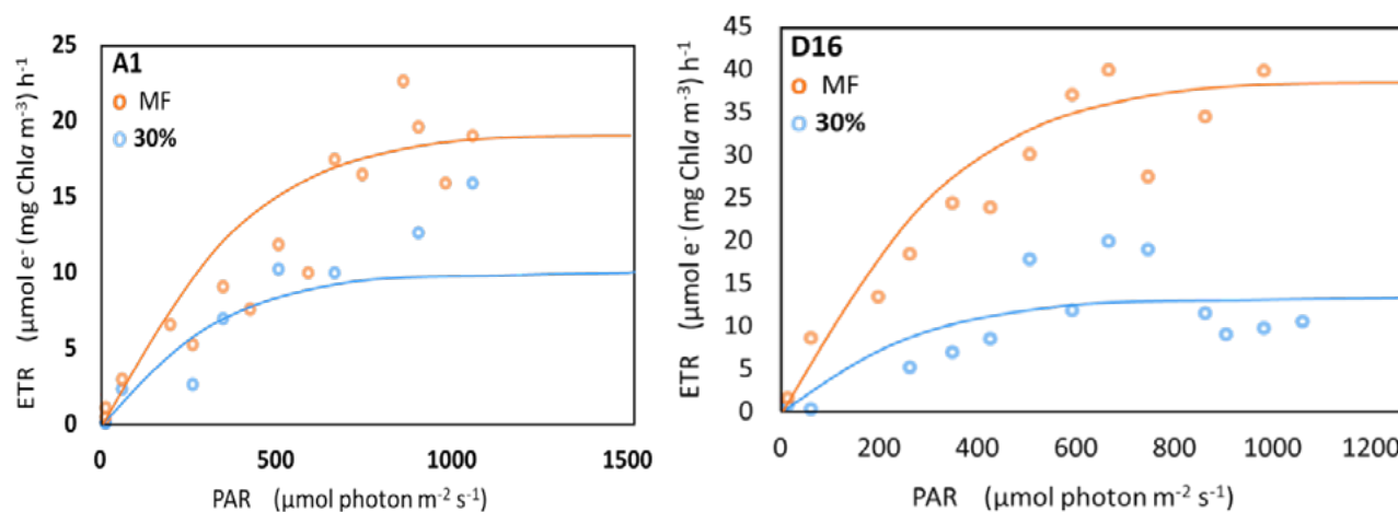
Figura 2. Curvas tasa de transferencia de electrones -Irradiancia (ETR-E) al 30% de E_0 y del Máximo de fluorescencia (MaxF), en la Región de Perdido (RP) estación A1 y en la Región de Coatzacoalcos (RC) estación D16, en el Golfo de México durante el crucero MMF-03.
