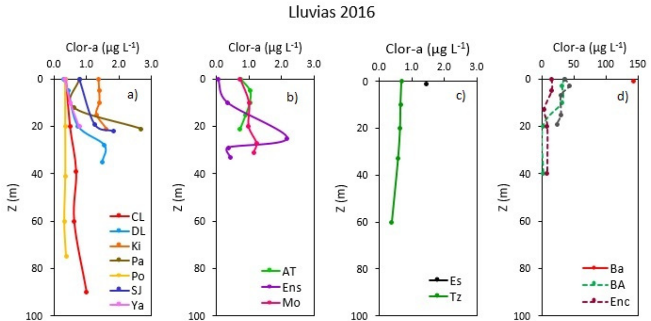
Figura 4. Distribución vertical de la Clor-a ( \mu\text{g L}^{-1} ) durante la temporada de lluvias 2016 en los lagos no impactados (a, b y c) e impactados (d) del PNLM.
