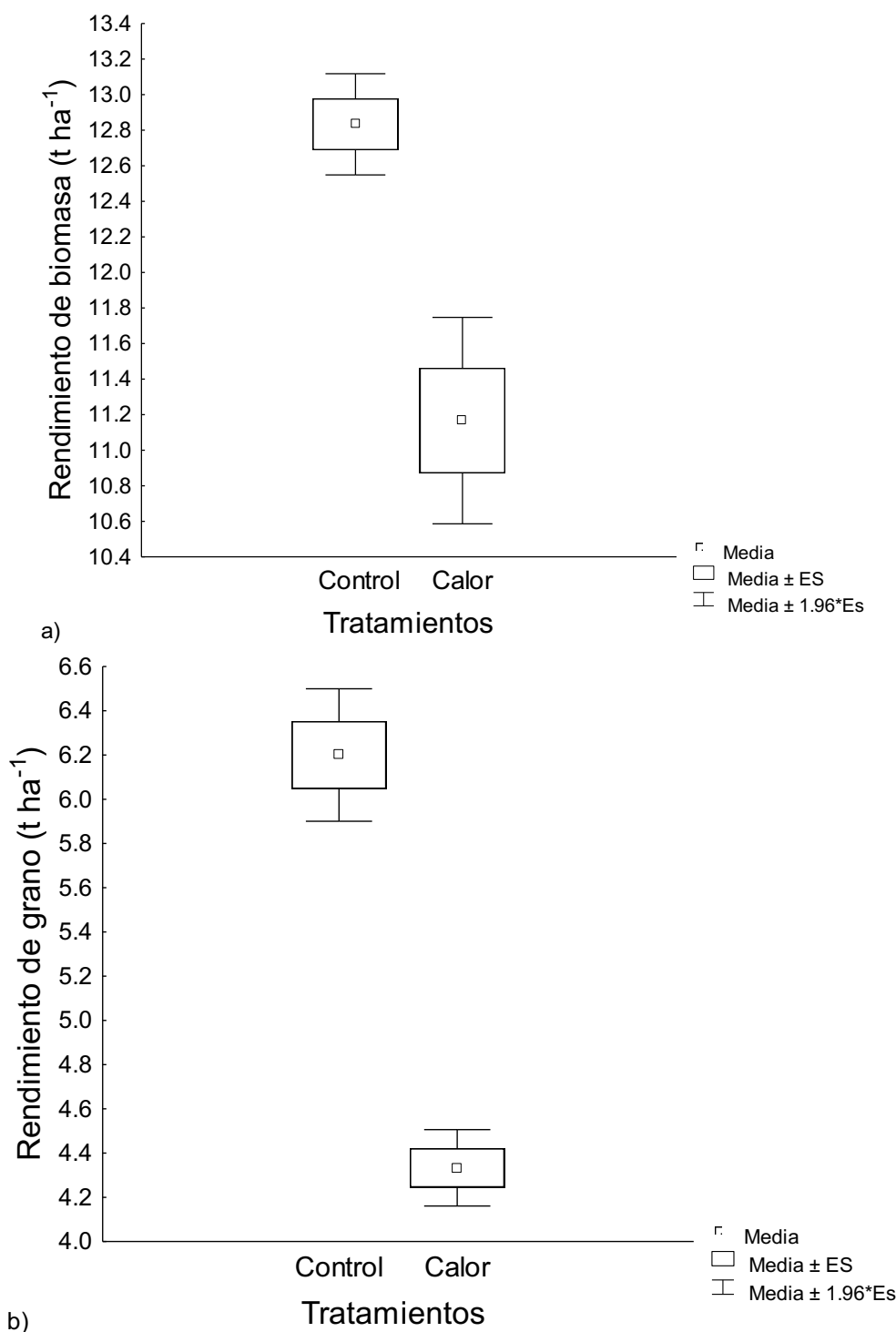
Figura 2. Rendimientos de biomasa (a) y de grano (b) de la variedad de trigo CIRNO C2008.
