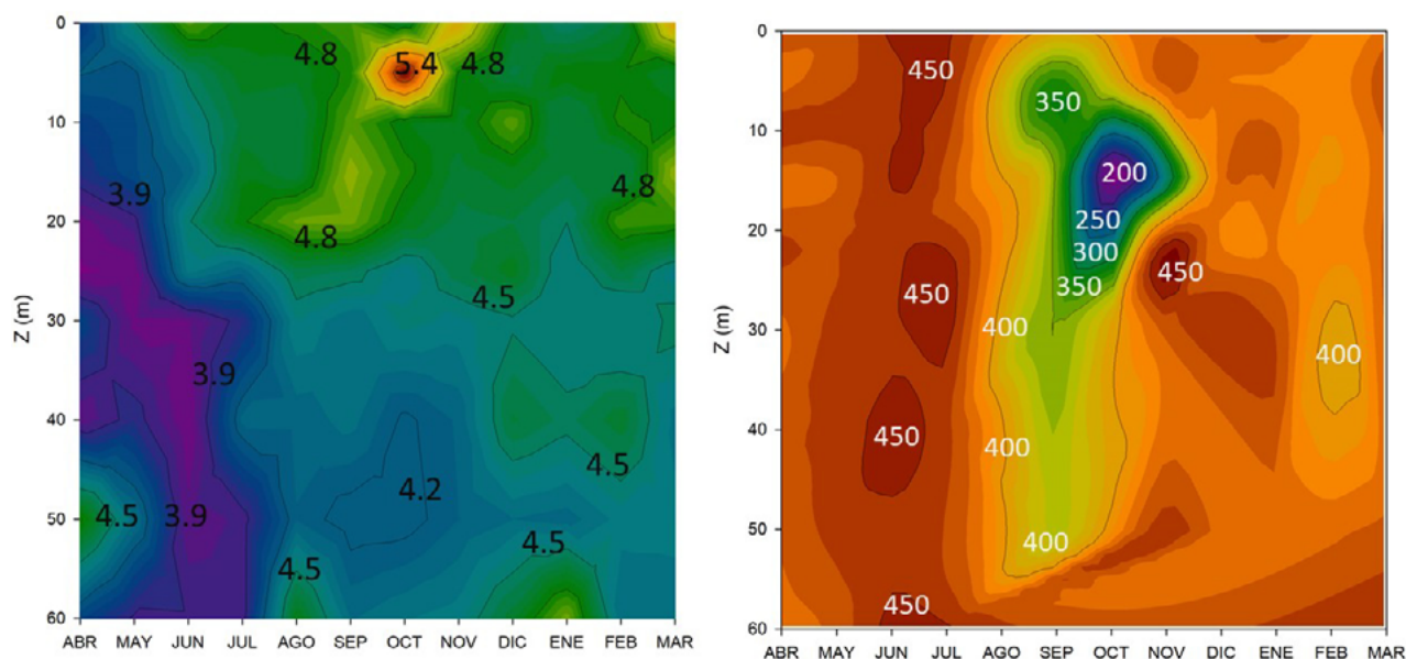
Figura 2. Variación de la concentración de COD (izq.) y CID (der.) en el perfil vertical del Lago Alchichica (2013-2014).
