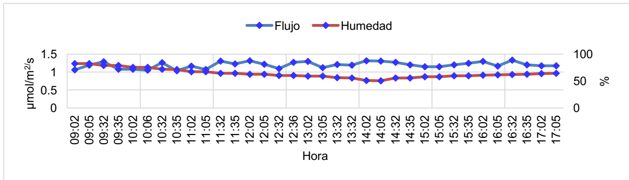
Figura 7. Flujo de CO 2 y humedad del suelo del sitio 3.
